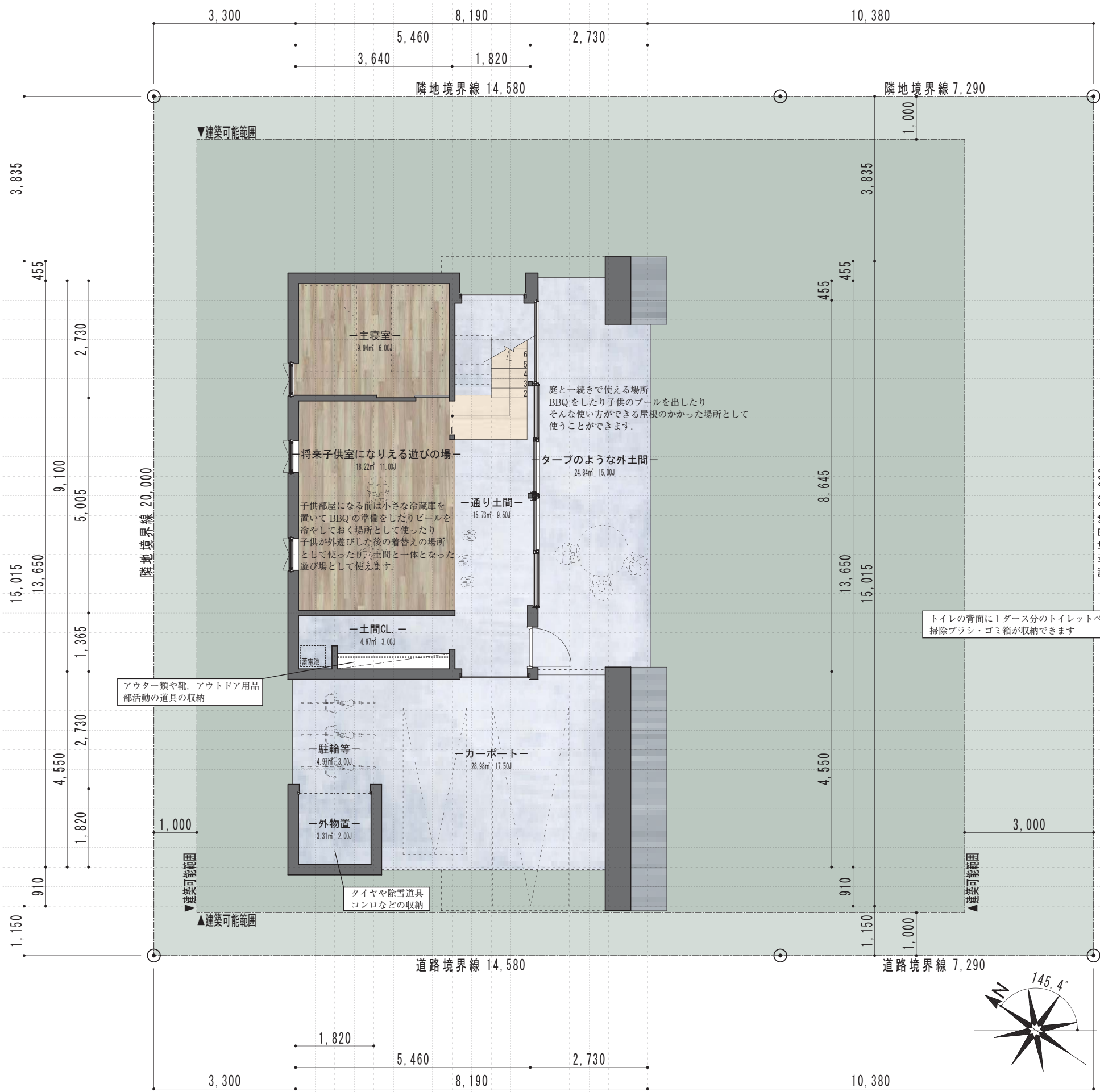
平面図 Scale 1/100
